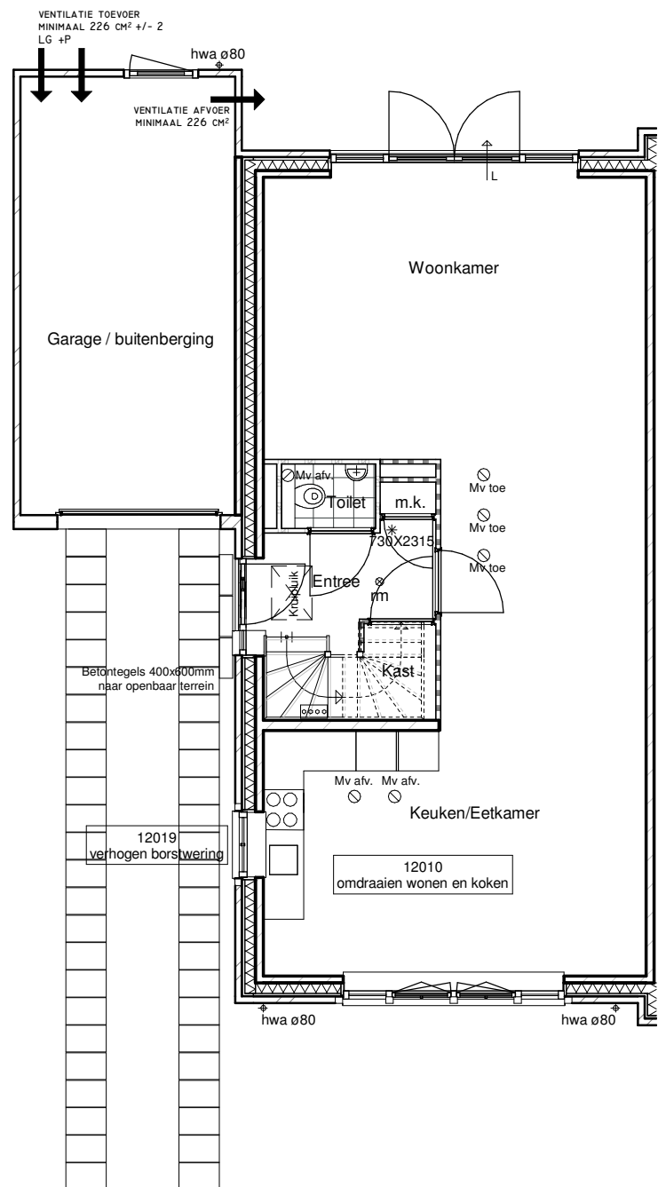
begane grond
